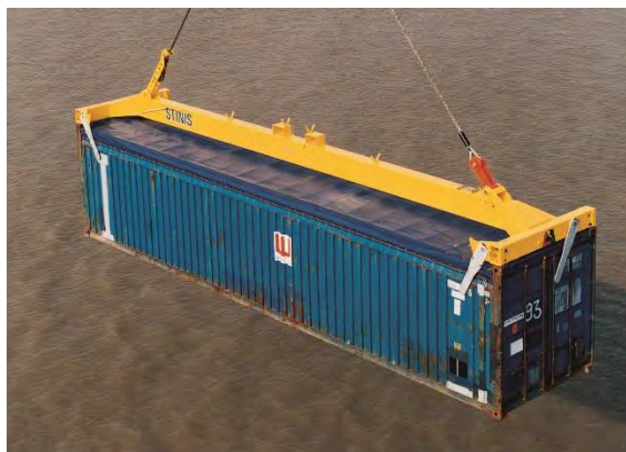
1989 STINIS AUTOTWIST®
