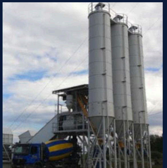
Бетоносмесительные установки (Германия)
